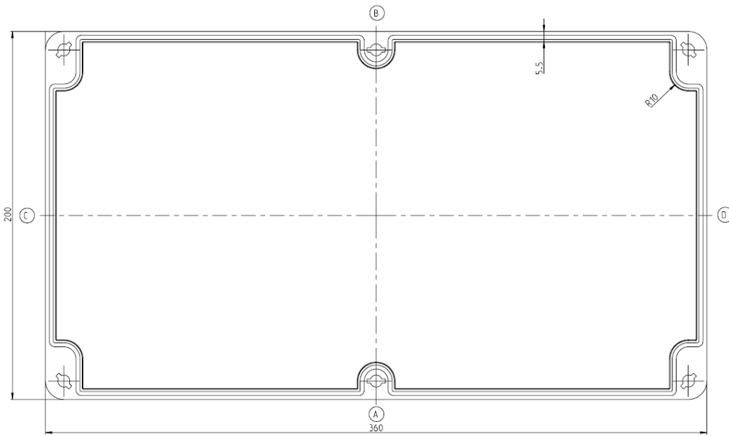
Lid
